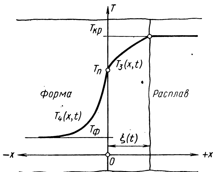
Рис. 30. Схема температурных полей к задаче С. Шварца для случая затвердевания неперегретого расплава
