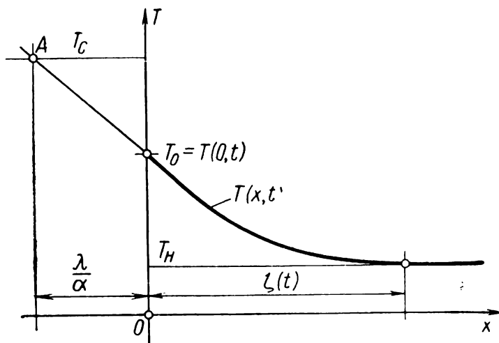
Рис. 10. Схема температурного поля в полуограниченном теле при нагреве его в соответствии с граничным условием III рода
