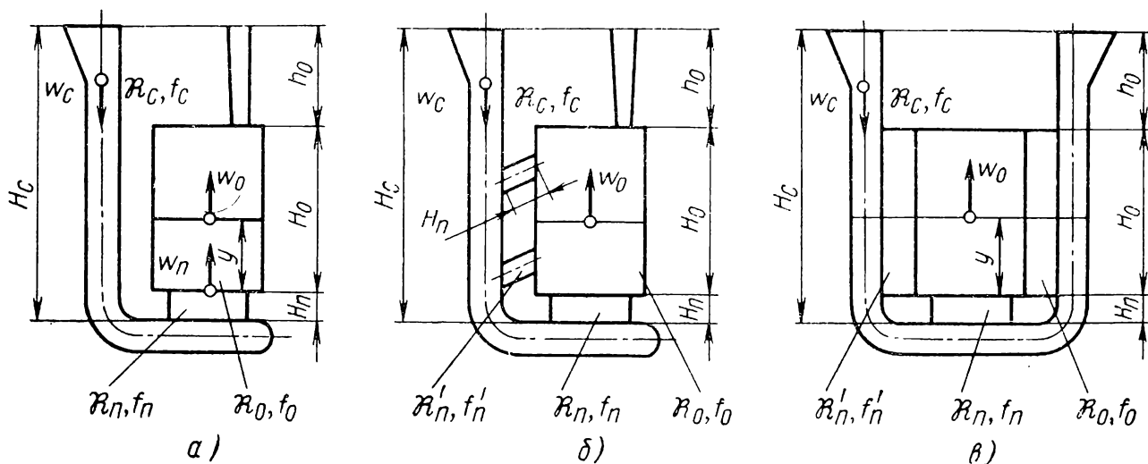
Рис. 69. Схема литниковых систем в кокилях:
