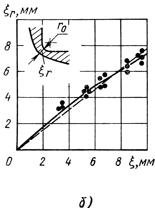
Рис. 46. Профиль затвердевающей корки (а), рассчитанной по формуле (102). Толщина корки (б) у внешнего угла формы с галтелью по данным Б. Б. Гуляева; кривая рассчитана по (103)
