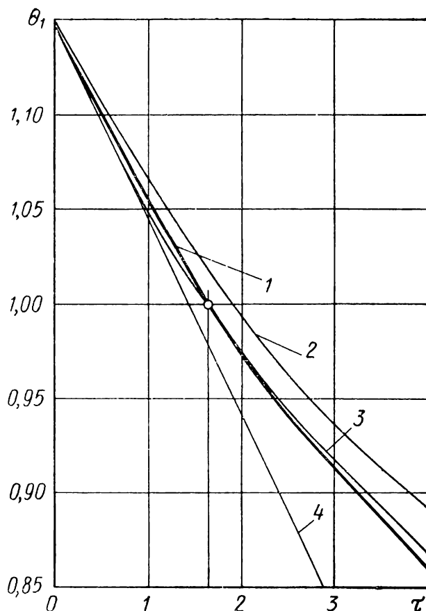
Рис. 67. Сопоставление результатов расчета: охлаждения перегретого расплава
