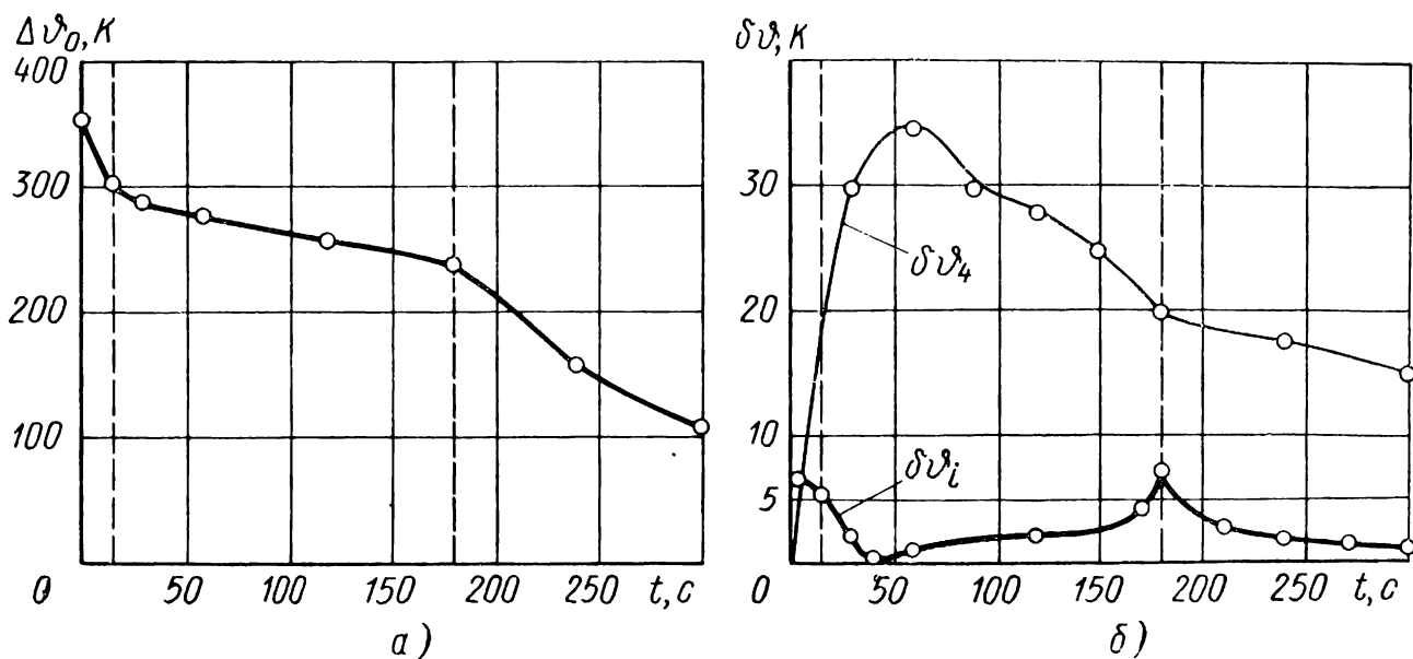
Рис. 63. Изменения температурного напора на границе контакта отливки и формы (а) и температурных перепадов в отливке и в форме (б) во время затвердевания цинка в кокиле
