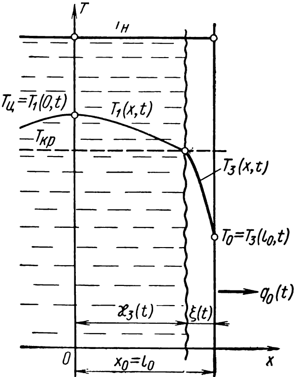
Рис. 20. Схема температурных полей в затвердевающей отливке из чистых металлов и эвтектических сплавов
