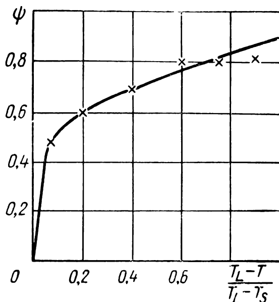
Рис. 50. Связь между относительным количеством твердой фазы и температурой расплава внутри интервала кристаллизации Бр.ОЦ 10-2
