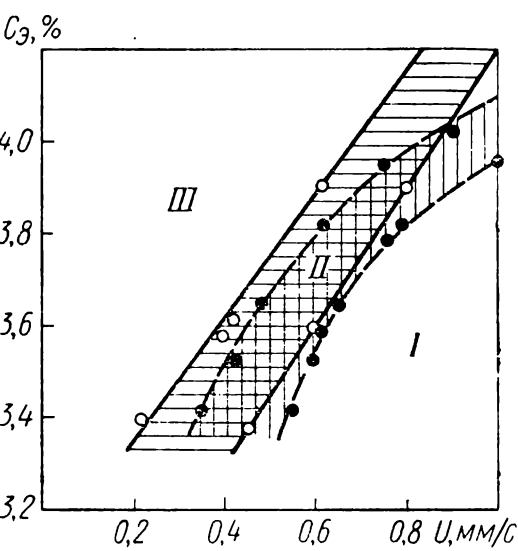
Рис. 16. Зоны белого (I), половинчатого (II) и серого перлитного (III) синтетических чугунов (при C/Si = 1,02 \div 1,25 ) в зависимости от углеродного эквивалента и скорости затвердевания отливок
