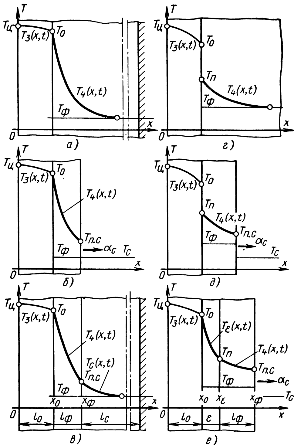
Рис. 25. Схемы температурных полей в отливке и форме:
