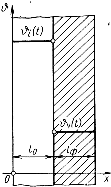
Рис. 64. Схема температурных полей в отливке и кокиле
