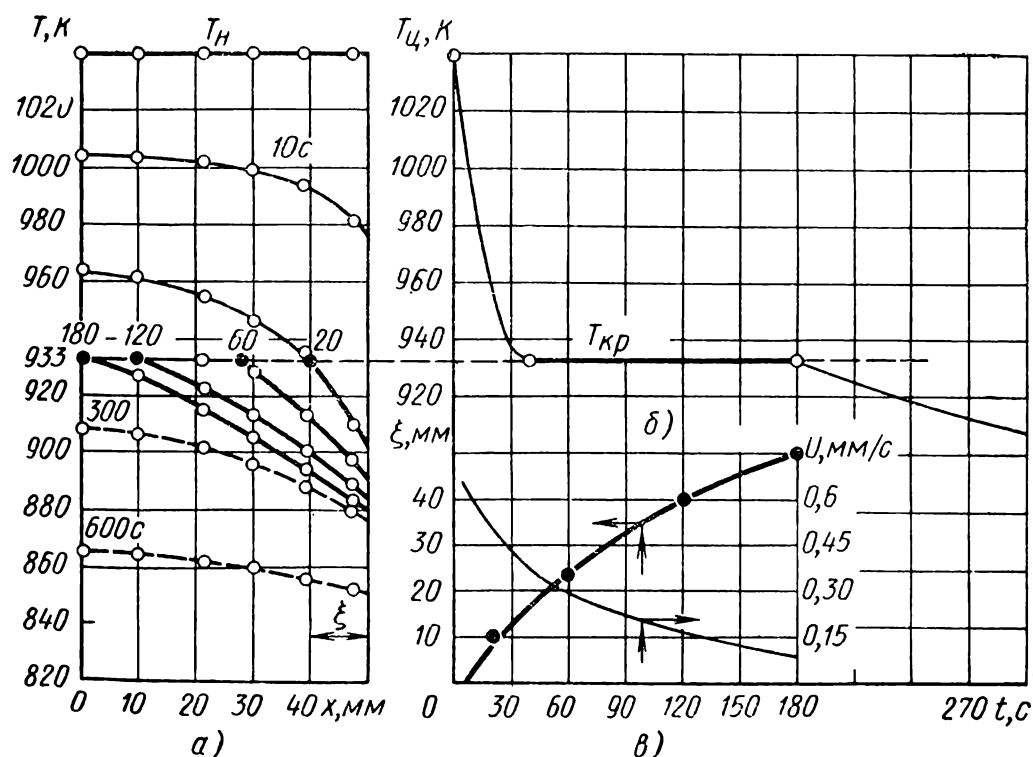
Рис. 19. Температурные поля (а), кривая охлаждения (б) и кинетика затвердевания (в) отливки из алюминия А0 в чугунном кокиле
