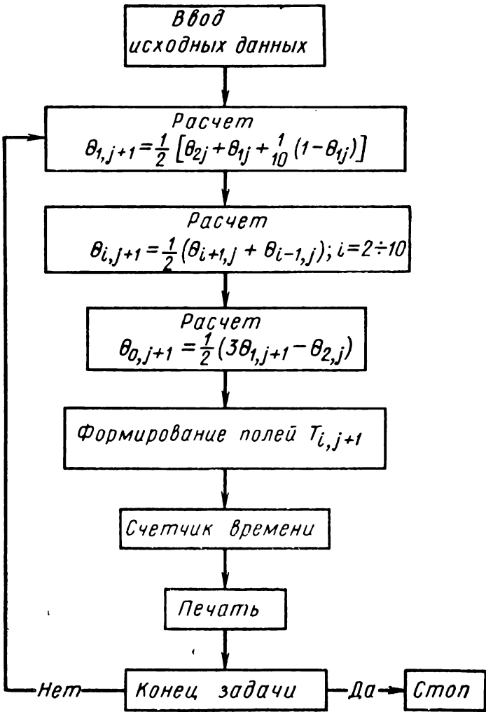
Рис. 11. Блок-схема численного расчета нагрева полубесконечного тела на ЭЦВМ
