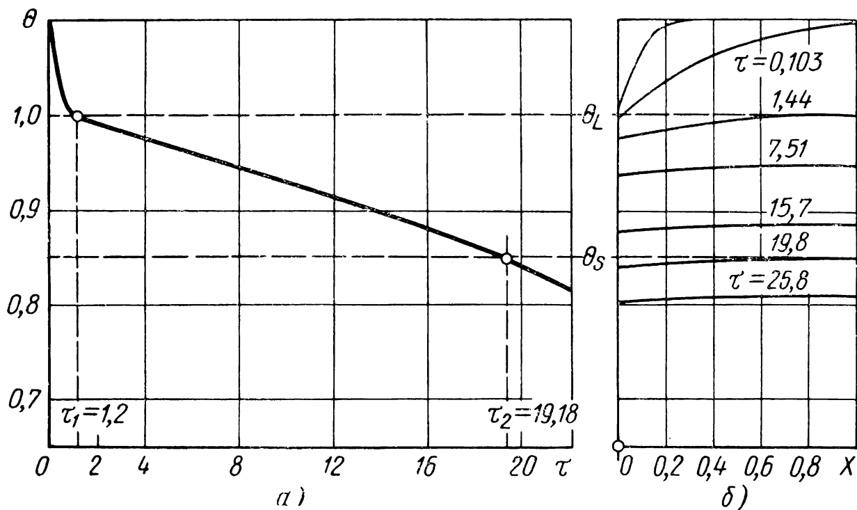
Рис. 51. Кривая охлаждения затвердевающего расплава (а) и температурные поля в затвердевающей отливке (б), построенные по результатам численного решения задачи (119)–(125)
