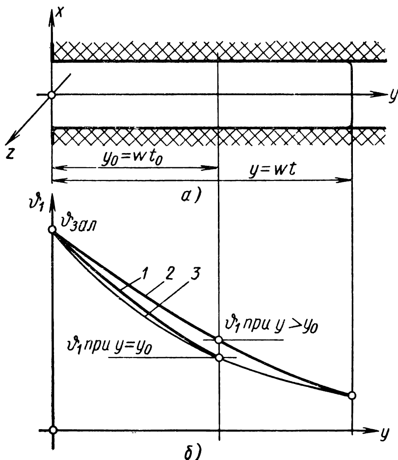
Рис. 38. Схема к анализу охлаждения потока перегретого расплава при его течении в горизонтальном щелевом канале песчаной формы:
