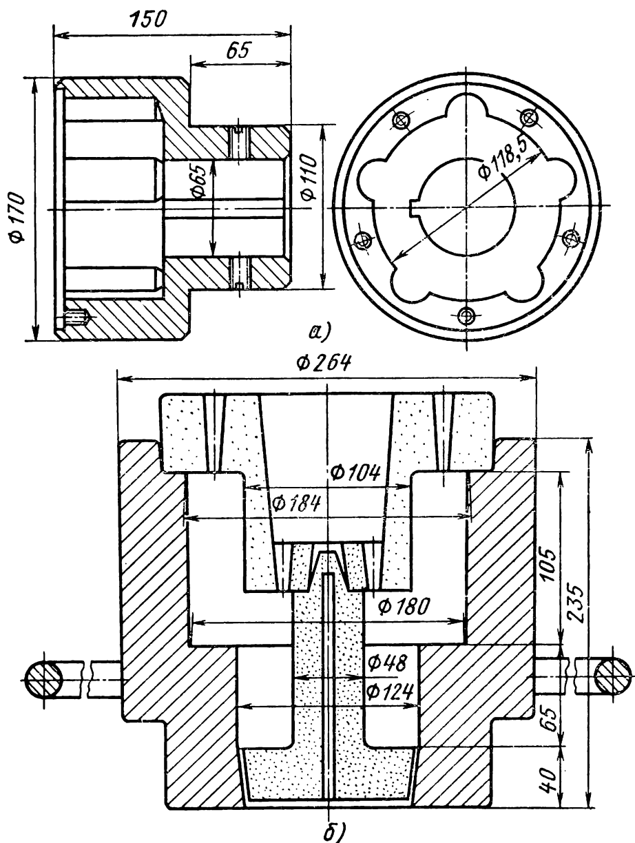
Рис. 71. Муфта (а) и продольный разрез кокиля для отливки муфты (б)
