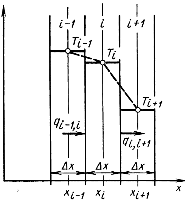
Рис. 6. Схема к выводу конечно-разностного уравнения охлаждения i -го слоя бесконечной плиты
