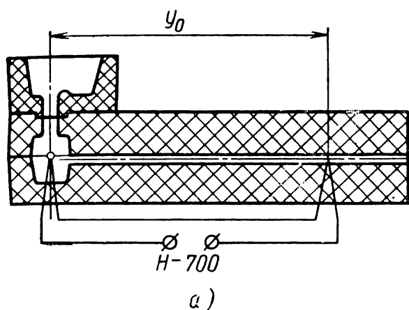
Рис. 39. Схема эксперимента (а) и результаты (б) измерения разницы температуры потока перегретого расплава в горизонтальном канале песчаной формы
