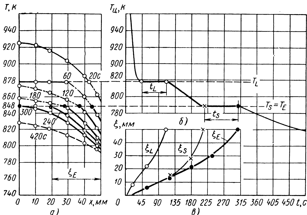
Рис. 24. Температурные поля (а), кривая охлаждения (б) и кинетика затвердевания (в) отливки из сплава алюминия, содержащего 7% Si, в чугунном кокиле
