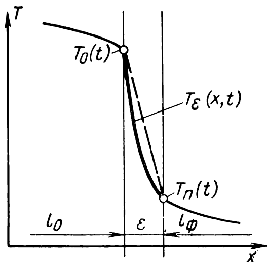
Рис. 26. Схема распределения температуры T_{\varepsilon}(x, t) по сечению слоя кокильной краски
