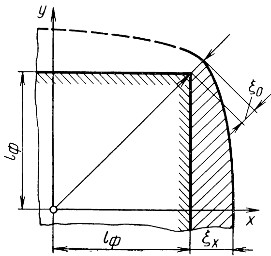
Рис. 70. Схема профиля твердой корки, затвердевающей у внешнего угла кокиля
