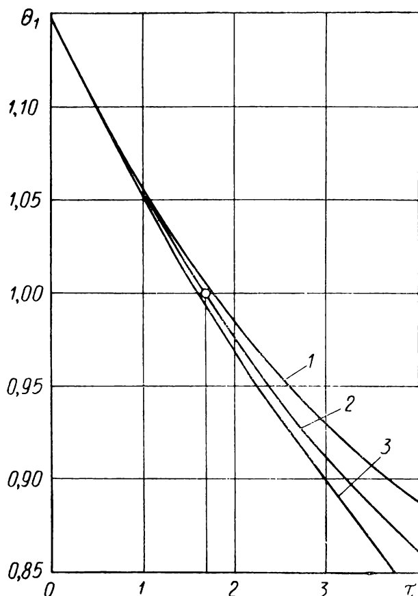
Рис. 66. Расчет охлаждения перегретого расплава по (40) при:
