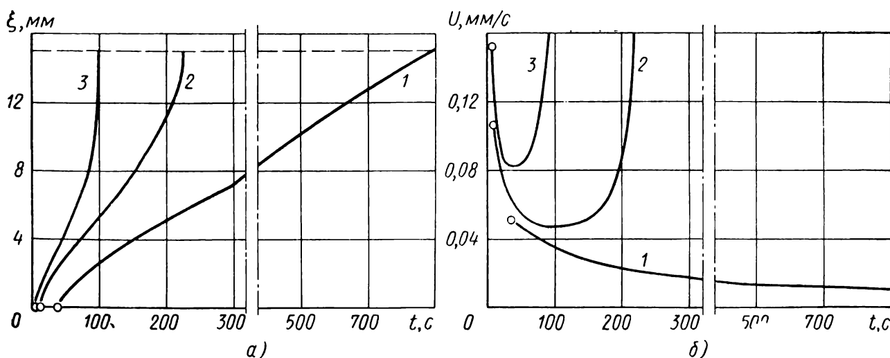
Рис. 43. Кинетика затвердевания (а) и изменения линейной скорости затвердевания (б) расплава силумина в форме для отливок:
