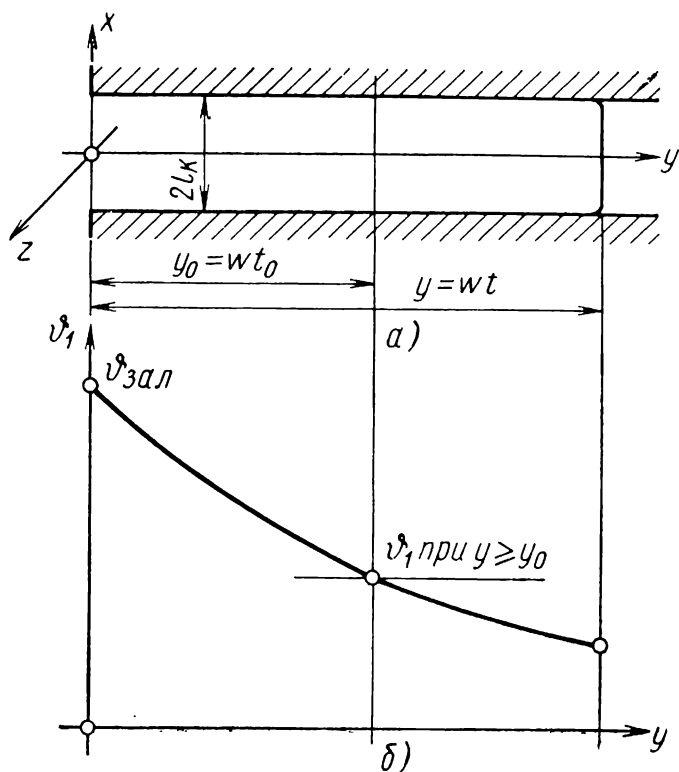
Рис. 68. Схема к анализу охлаждения потока перегретого расплава при его течении в горизонтальном канале:
