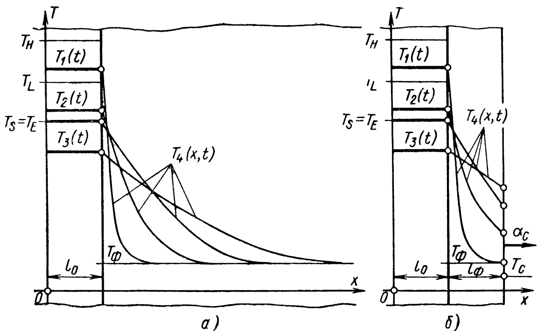
Рис. 32. Схемы температурных полей в отливке и формах:
