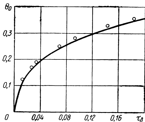
Рис. 12. Изменение температуры поверхности полуограниченного тела при нагреве его в соответствии с граничным условием III рода. Кривая рассчитана по (98), точки — по (100) и (101) при X_\delta = 0 и n = 2
