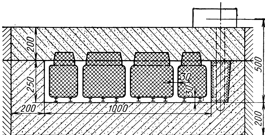
Рис. 61. Схема продольного разреза формы для отливки стола фрезерного станка
