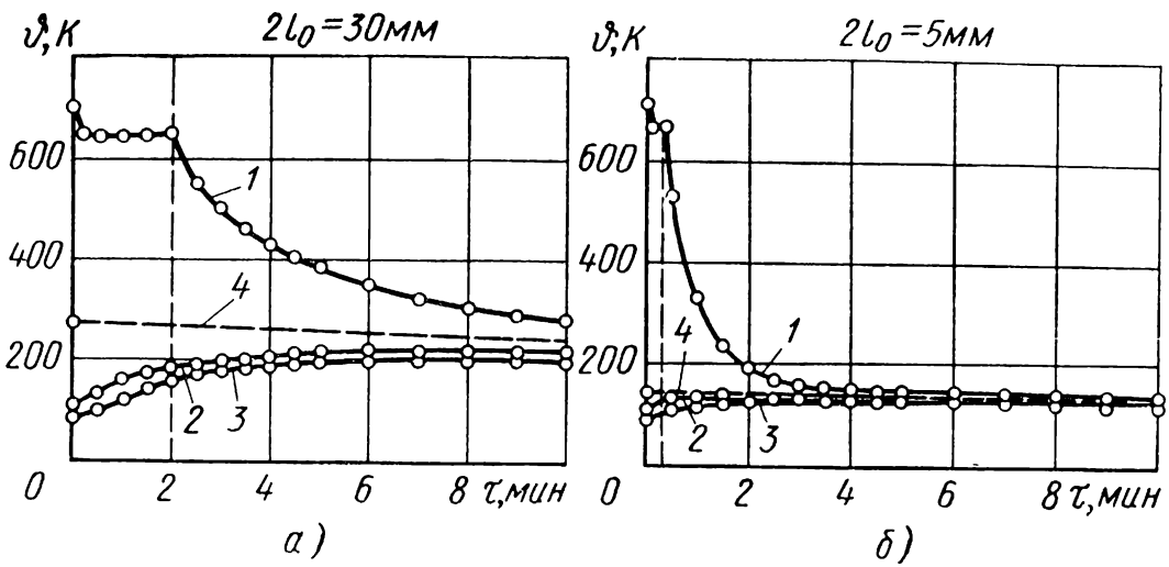
Рис. 65. Кривые изменения температуры центра (1) алюминиевой отливки, внутренней (2) и наружной (3) поверхностей кокиля и средней калориметрической температуры системы отливка—кокиль (4) во время затвердевания и охлаждения отливки при:
