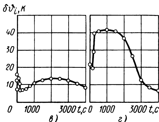
Рис. 28. Температурные поля ( а, б ) и температурные перепады ( в, г ) в чугуновой ( а, в ) и стальной ( б, г ) отливках, затвердевающих в сухой песчаной форме
