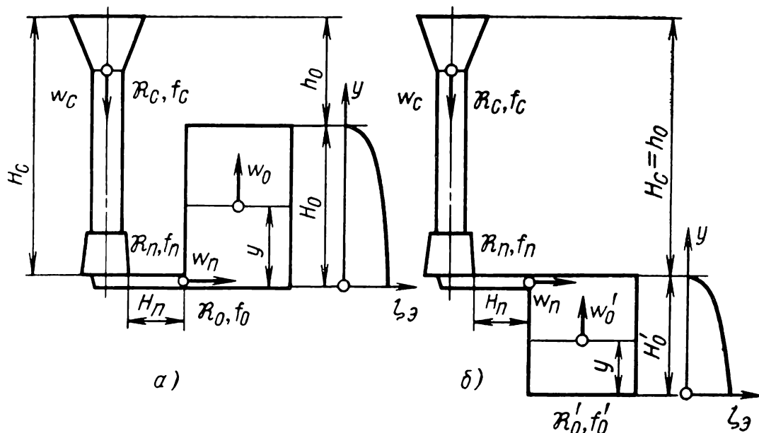
Рис. 40. Схема к расчету заполнения полости формы сифоном (а) и сверху (б) в разъем формы
