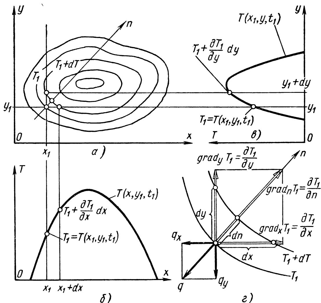
Рис. 2. Схема температурного поля в двумерном пространстве:
