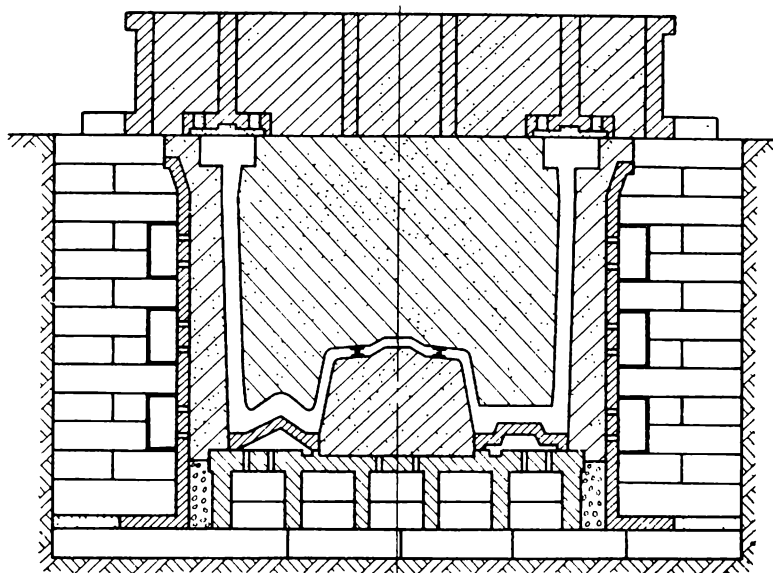
Рис. 60. Формовка станины продольно-строгального станка в охлаждаемом кессоне
