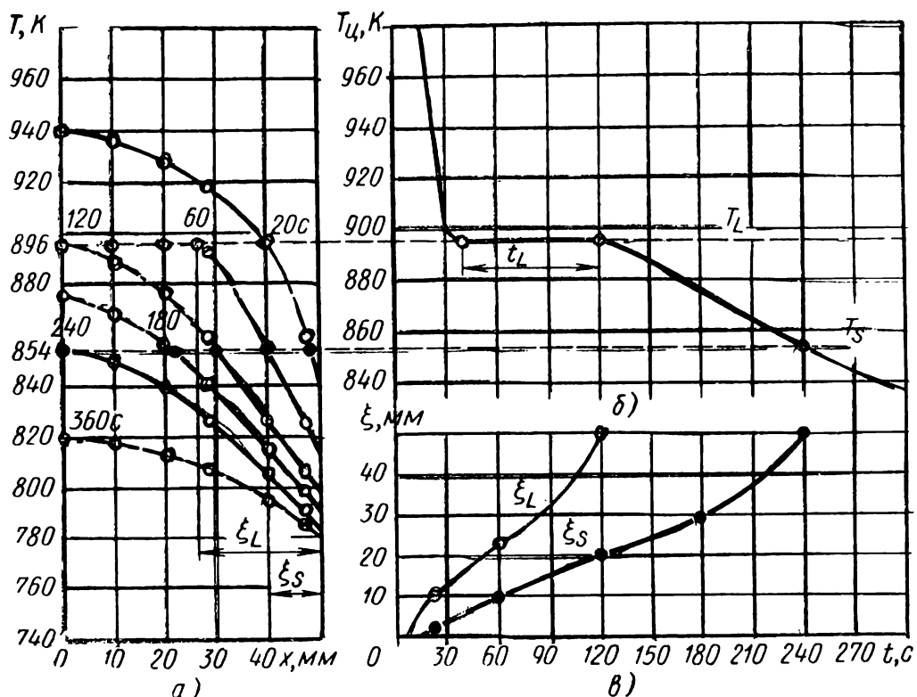
Рис. 21. Температурные поля (а), кривая охлаждения (б) и кинетика затвердевания (в) отливки из сплава алюминия, содержащего 20% Zn, в чугунном кокиле
