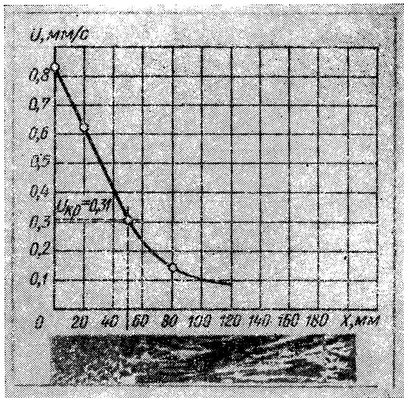
Рис. 17. Зависимость кристаллического строения слитка из сплава алюминия, содержащего 3% Si, от скорости его затвердевания при односторонне направленном отводе теплоты
