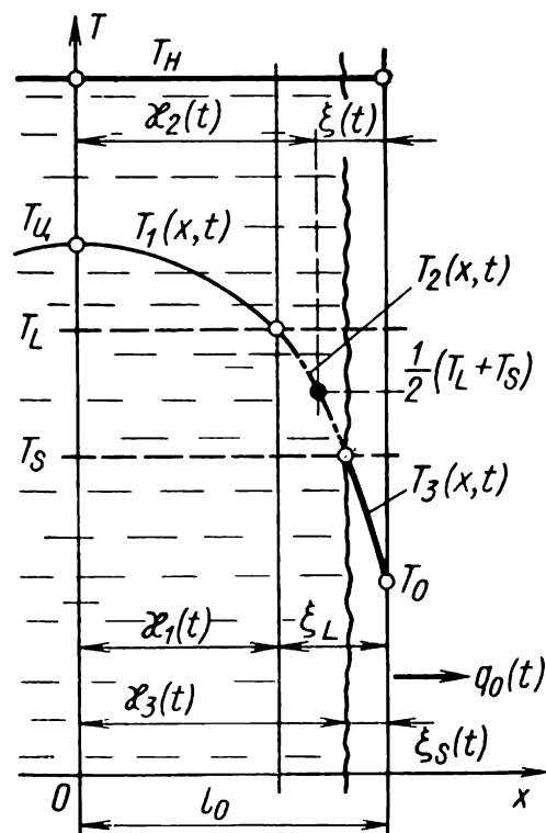
Рис. 22. Схема температурных полей в затвердевающей отливке из сплавов типа твердых растворов
